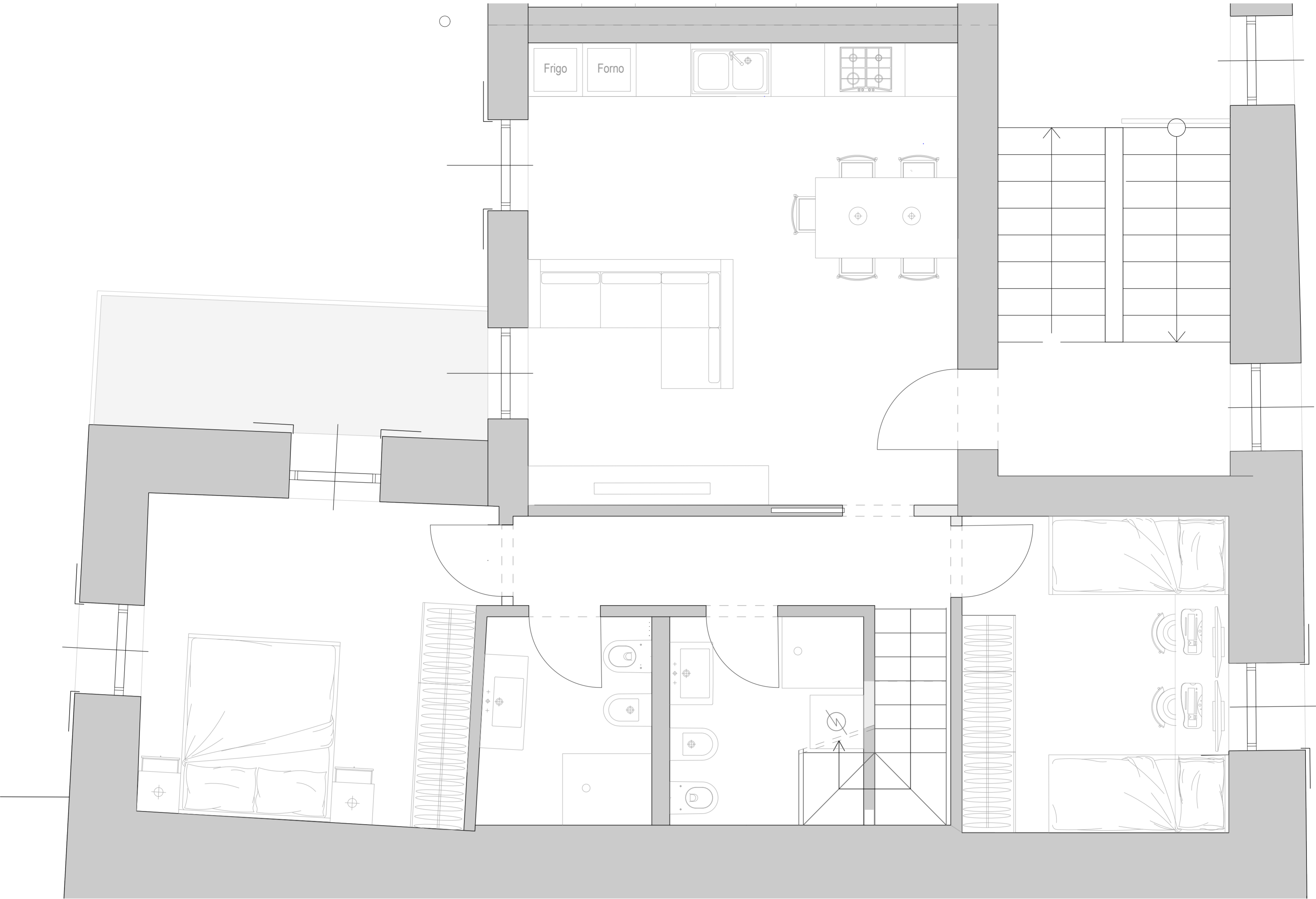
PIANTA PIANO TERZO-Appartamento 3
