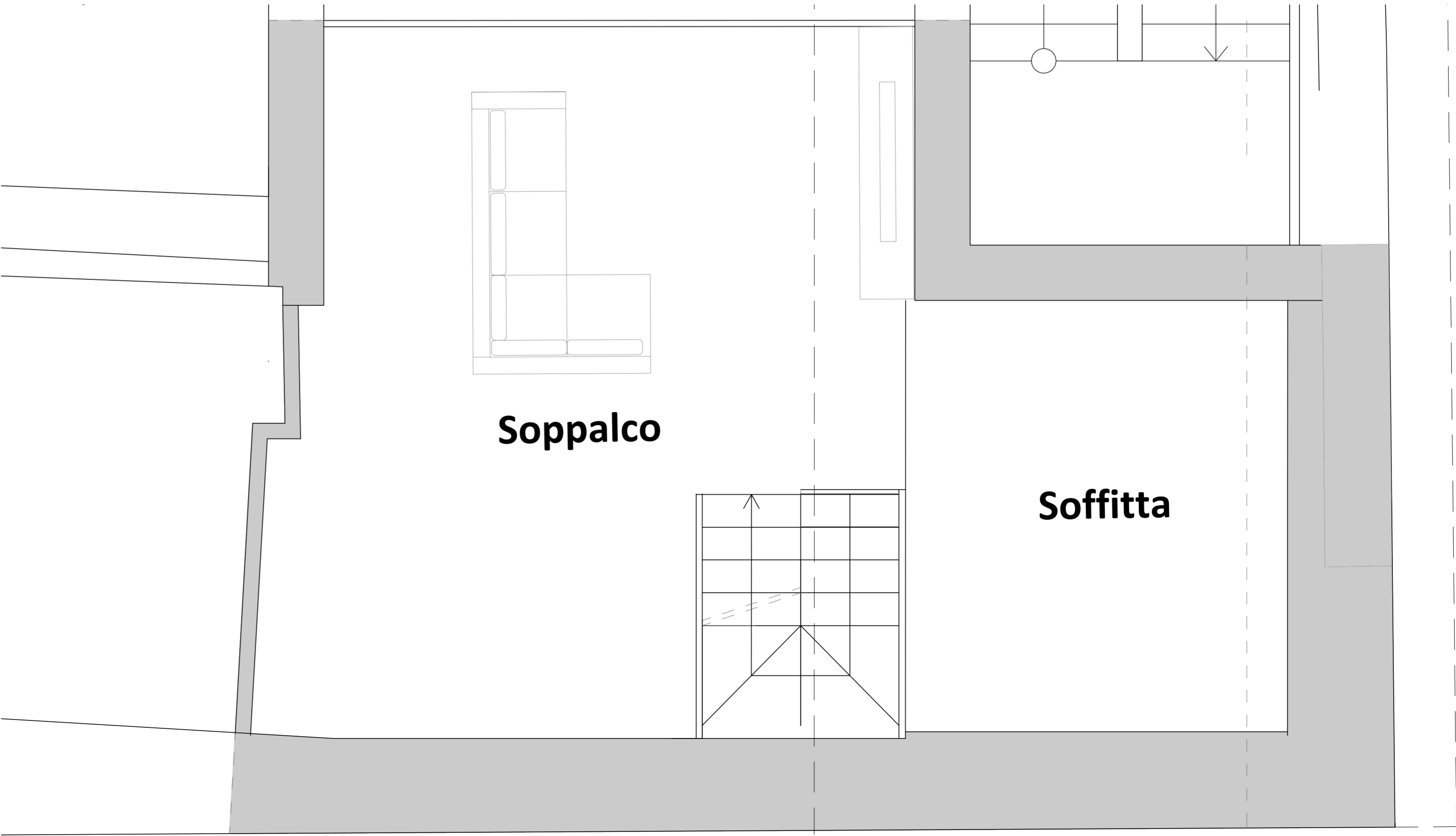
PIANTA PIANO TERZO-Appartamento 3
